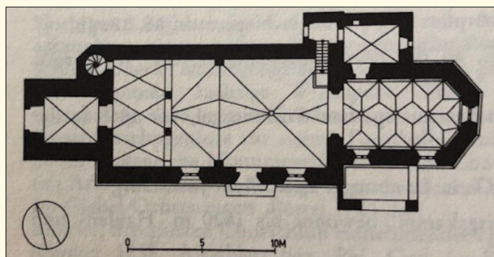
Abb.: Grundriss vor 1976 - Entfernung von Kanzel und Zubau für Kriegerdenkmal
